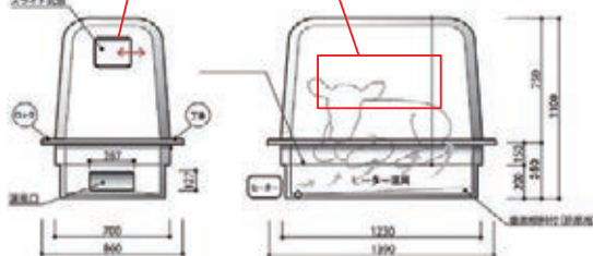
のぞき窓 (550×250)
